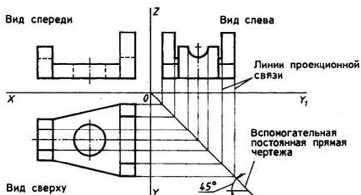
Рис. 2. Построение третьей проекции по двум заданным с помощью постоянной прямой чертежа
